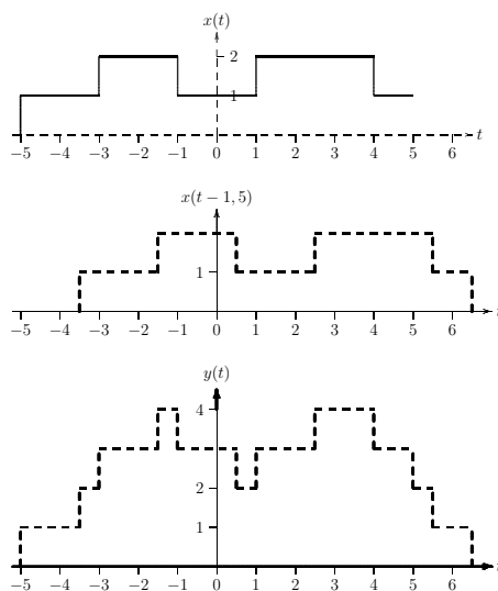
Figur 1: Exempel på dispersion. y(t) = x(t) + x(t - 1.5)
