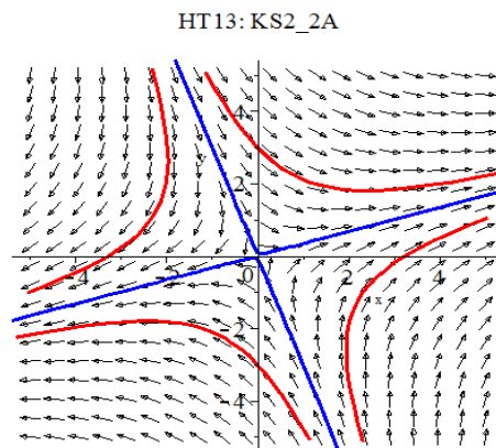
Figur 1: x' = 4x + 3y, y' = 3x - 4y
