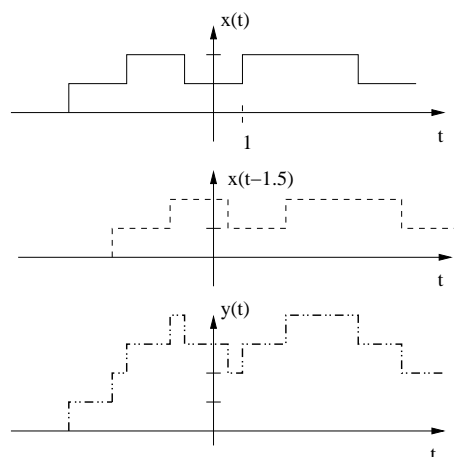
Figur 1: Exempel på dispersion. y(t) = x(t) + x(t - 1.5)
