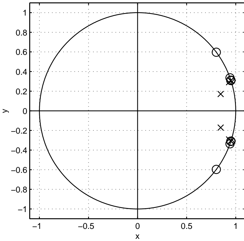
Pol-Nollst-Diagr av LP-filtret
