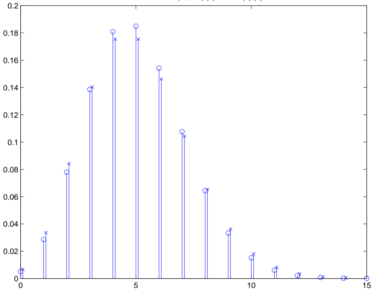
Jämförelse Bin(50,0.1) (o) och Po(5) (x)
