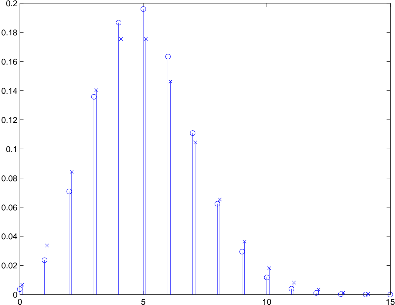
Jämförelse Bin(25,0.2) (o) och Po(5) (x)
