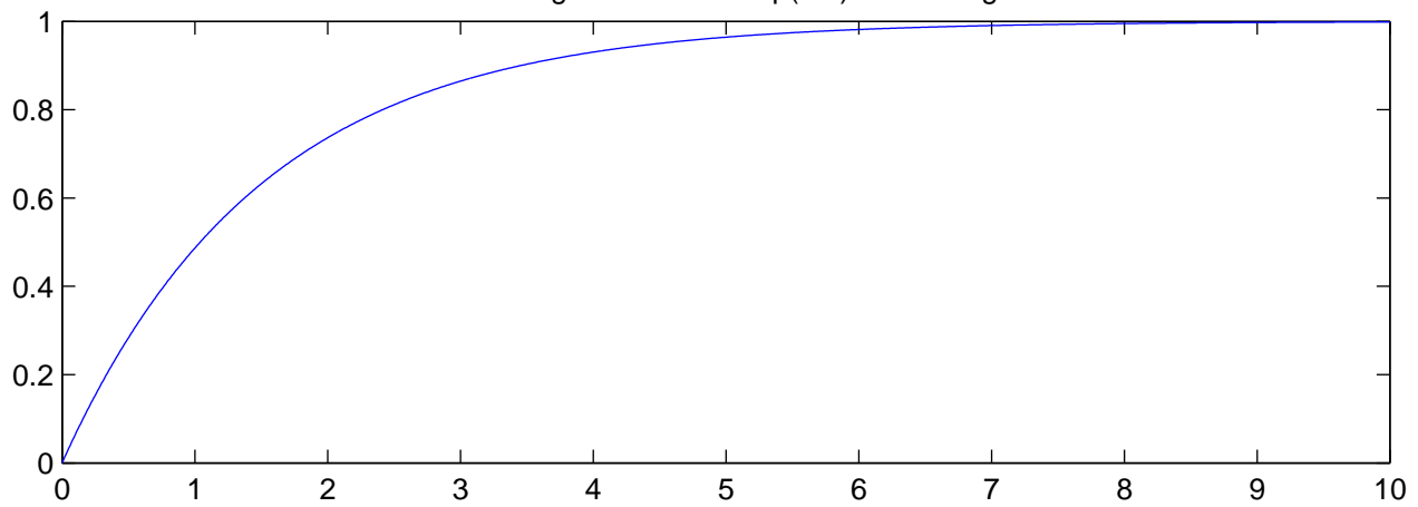
Fördelningsfunktion för Exp(1.5)-fördelningen
