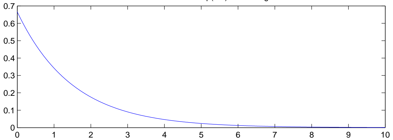
Täthetsfunktion för Exp(1.5)-fördelningen
