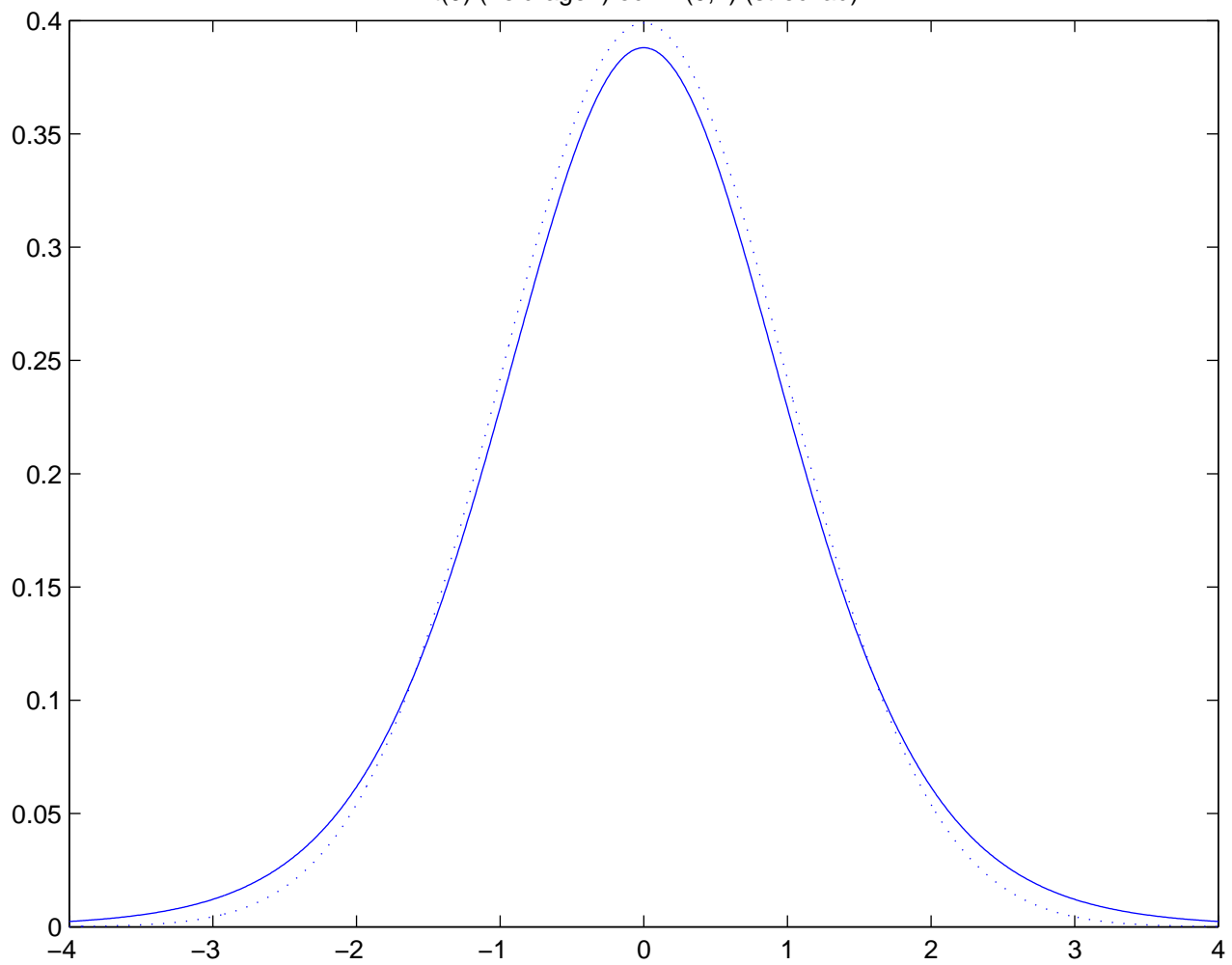
t(9) (heldragen) och N(0,1) (streckad)
